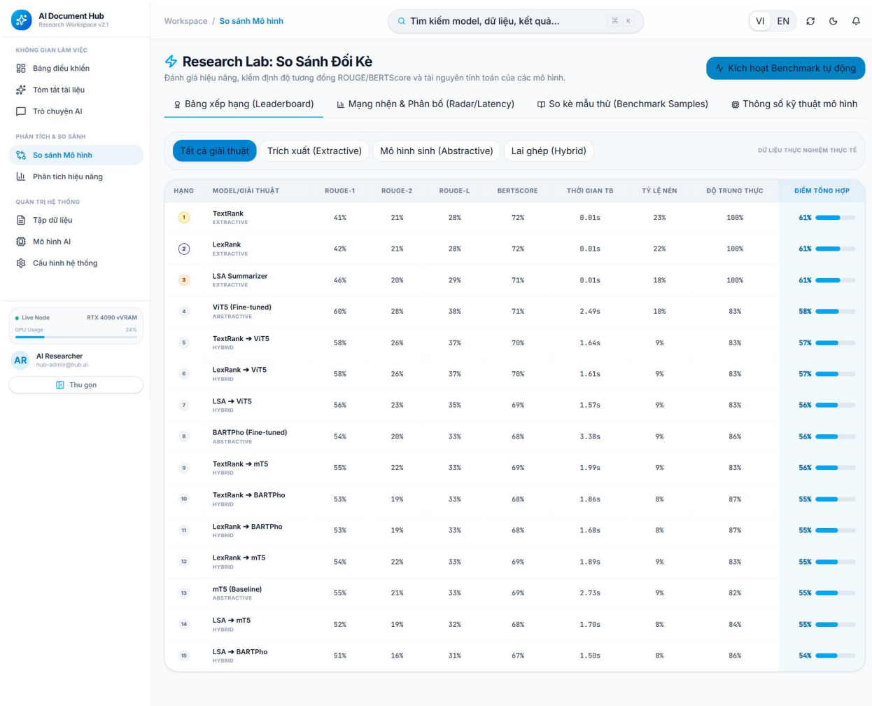
Hình 3.5. Giao diện đánh giá kết quả
