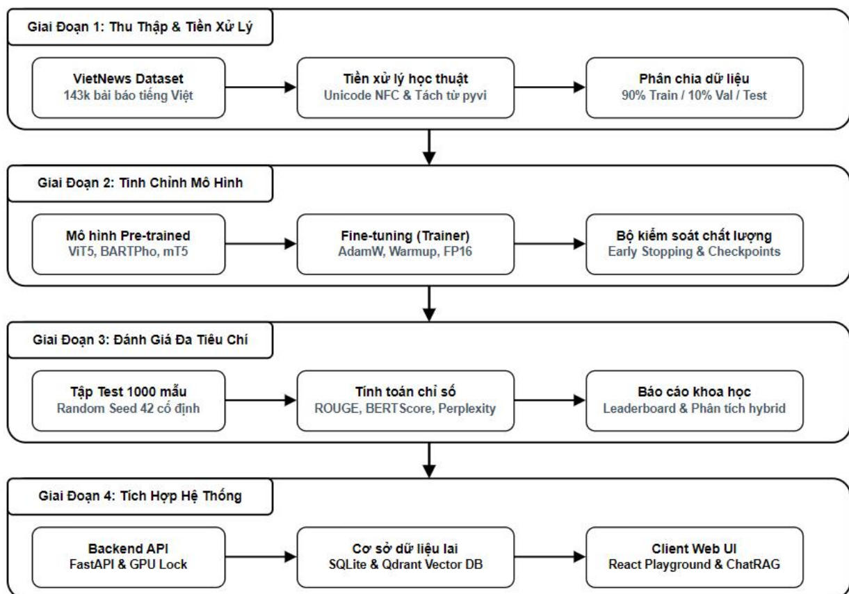
Hình 3.6. Sơ đồ kiến trúc nghiên cứu
