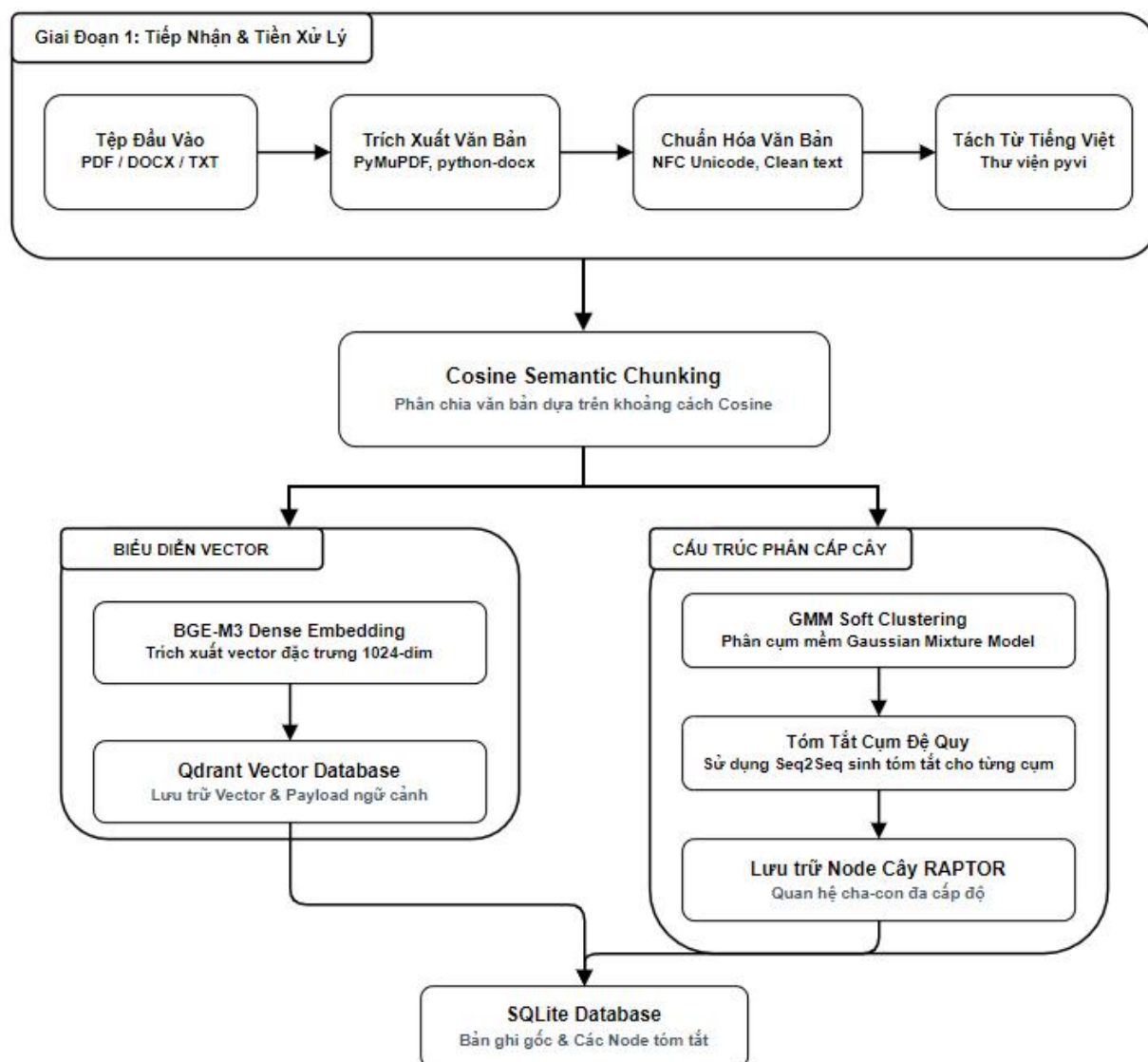
Hình 3.7. Sơ đồ pipeline xử lý dữ liệu
