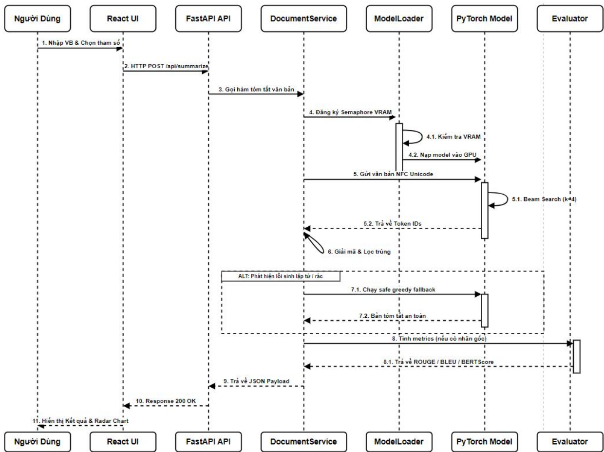
Hình 3.8. Sơ đồ tuần tự suy luận của mô hình
