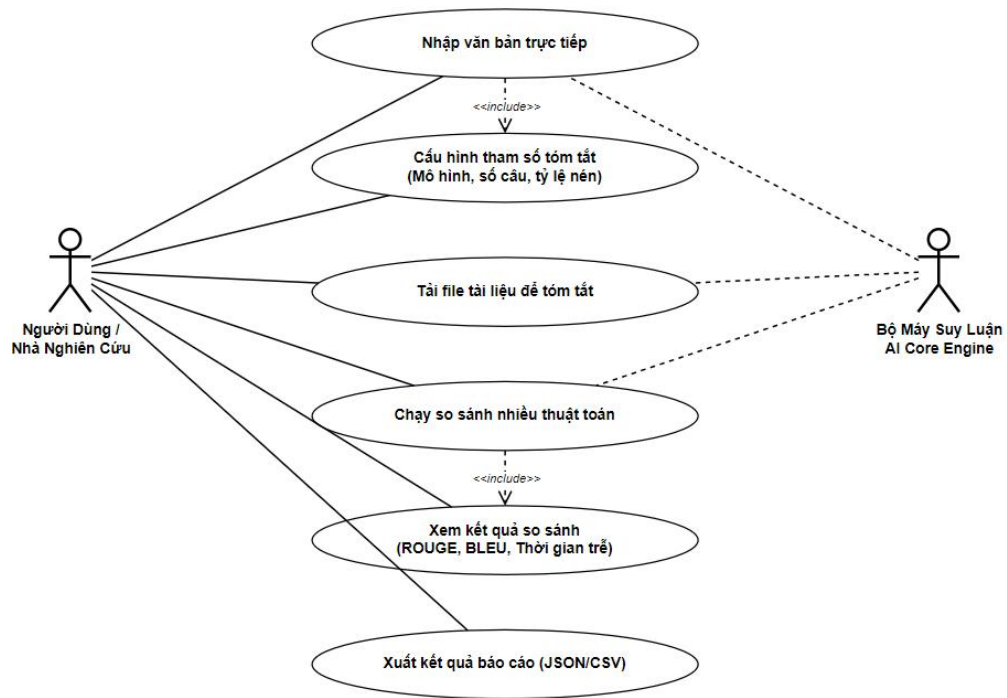
Hình 3.10. Sơ đồ Use case tóm tắt văn bản
