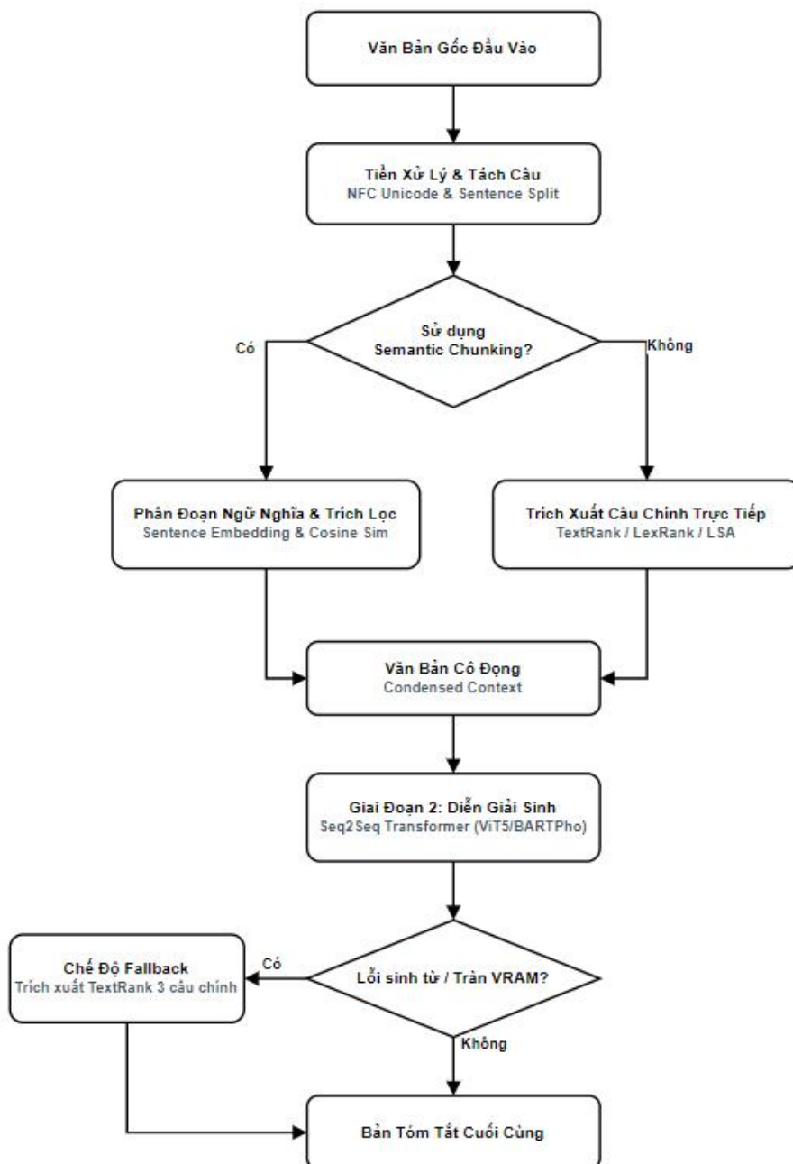
Hình 4.1. Sơ đồ pipeline tóm tắt Lại hai giai đoạn
