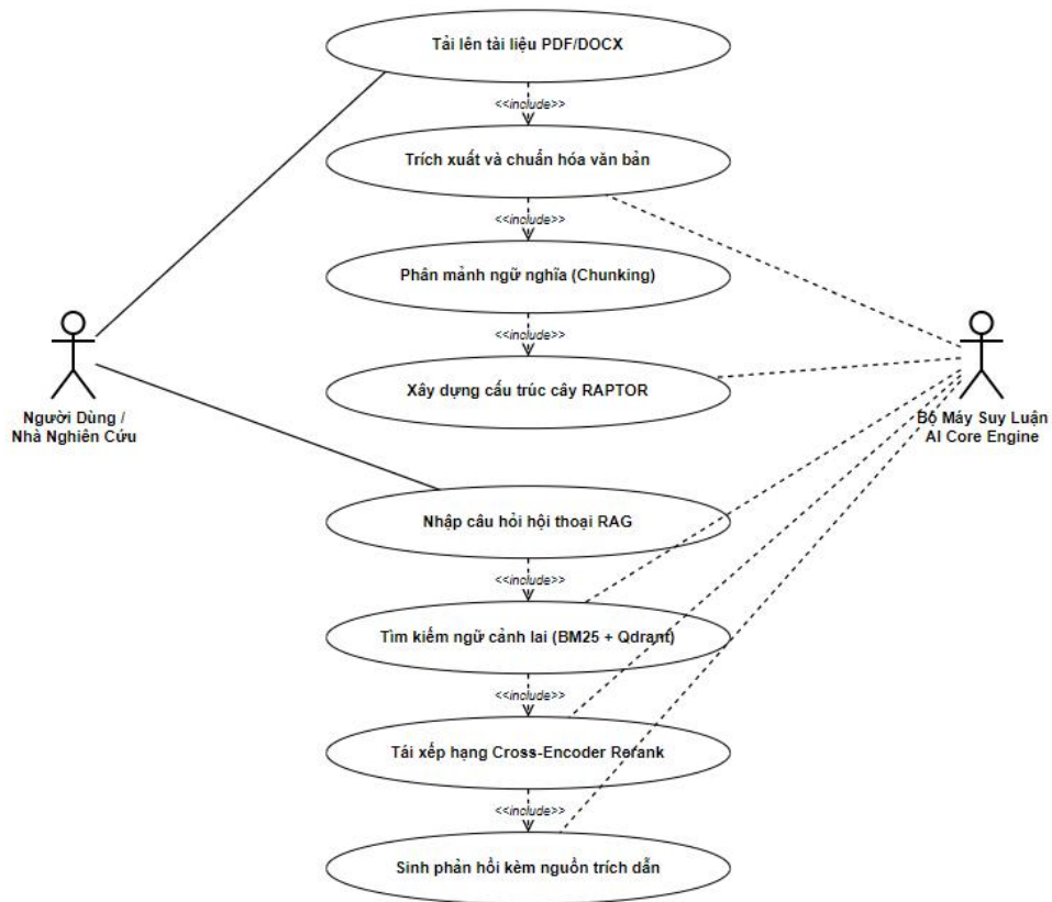
Hình 3.11. Sơ đồ Use case chatbot RAG
